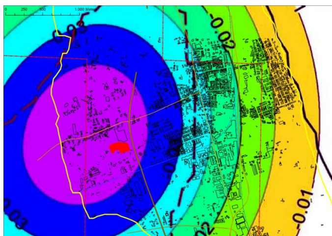
Fig.10: subsidenza stimata dal progetto di stoccaggio (in metri); in nero gli edifici di Porto d'Ascoli
